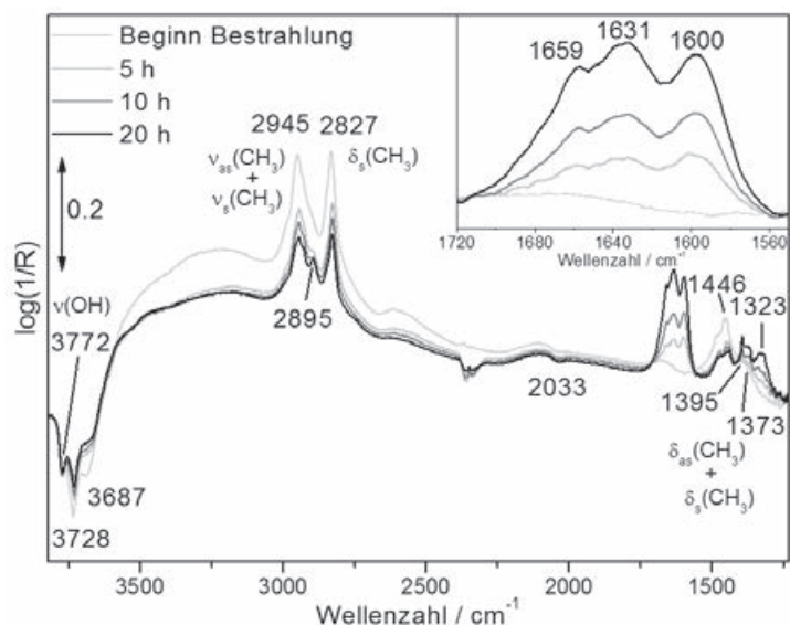
(8) In-situ-DRIFT-Spektren der Oxidation von Methanol an \text{V}(1.3)/\text{Al}_2\text{O}_3 -I. Die Bestrahlung der Probe erfolgte direkt in der IR-Messzelle mit einer 150\text{ W} Xe-Lampe über einen Lichtleiter.
