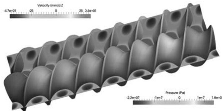
(19) Beispiel für die Simulation eines Doppelschraubenextruders.
