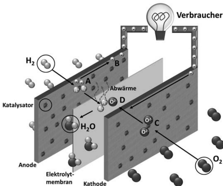
(1) Prinzipskizze einer Brennstoffzelle. Quelle: Zentrum für Brennstoffzellentechnik
