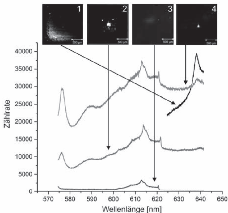
(4) Übersichtskarte eines 2x2 mm 2 Diamant (500x500 px). Der Kontrast ist durch die Zählrate des NV0 ZPL bei 575 (2-4) nm oder NV- ZPL bei 637 nm (1) gegeben. Die Spektren wurden vom Pixel mit der höchsten Intensität genommen.
