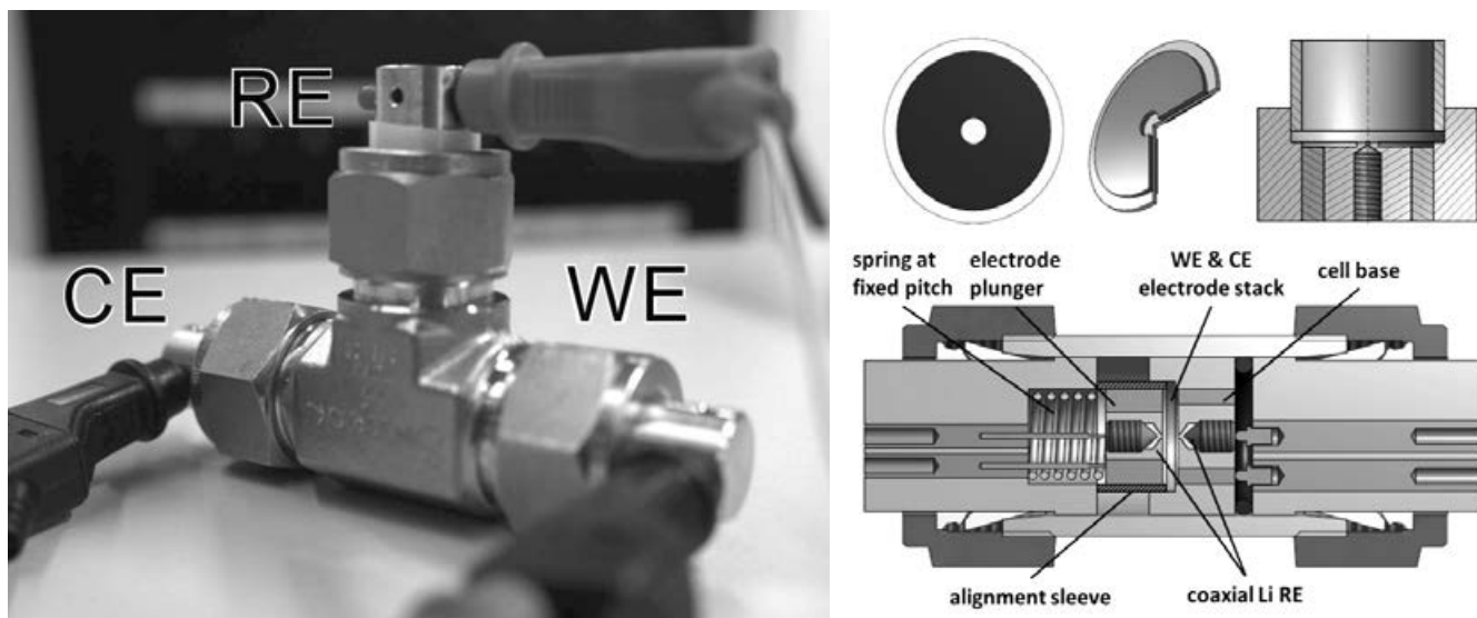
(5) Testzelle für elektrochemische Charakterisierungen. Links: klassische Swagelok® T-Zelle; rechts: Schema einer Messzelle mit koaxialer Referenzelektrode.
