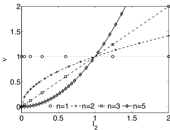
(12) Darstellung der Viskositätsfunktion für verschiedene Fließindizes n . Dilatanz (links) und Strukturviskosität (rechts).
