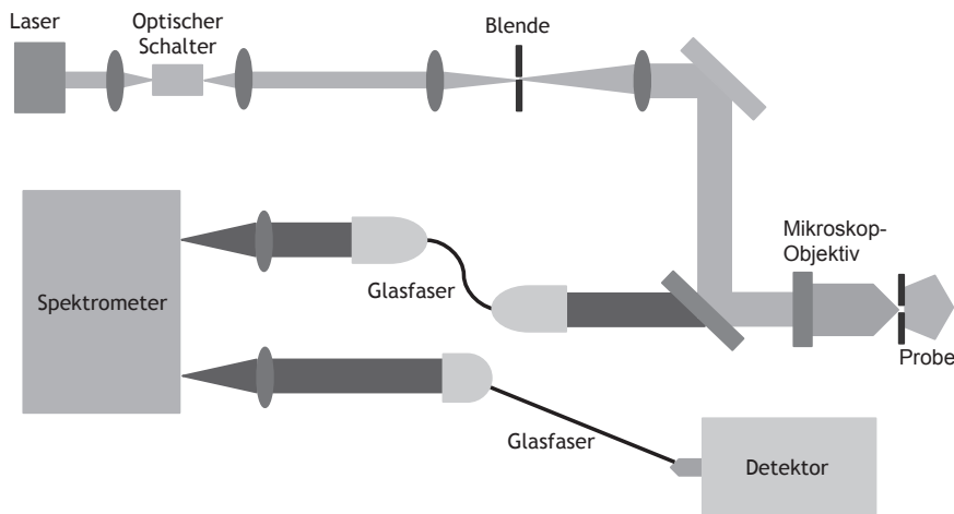
(6) Skizze des experimentellen Messaufbaus für die optisch detektierte magnetische Resonanz an einzelnen NV-Zentren.
