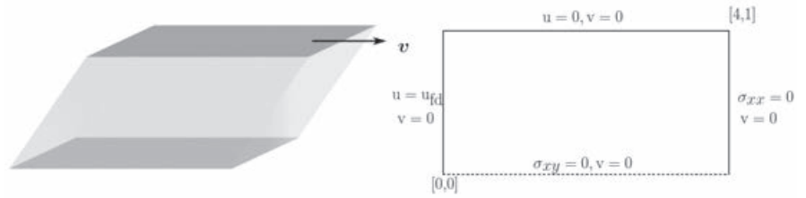
(13) Darstellung des numerischen Beispiels für eine Nicht-Newtonsche Fluid-Strömung zwischen zwei Platten.
