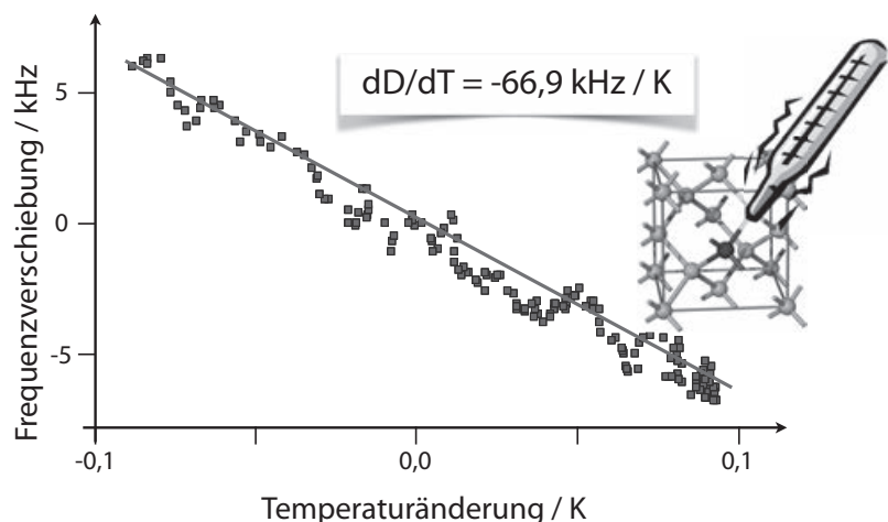
(7) Messung der Verschiebung der Resonanzfrequenz an einem einzelnen NV-Zentrum durch Temperaturänderung.
