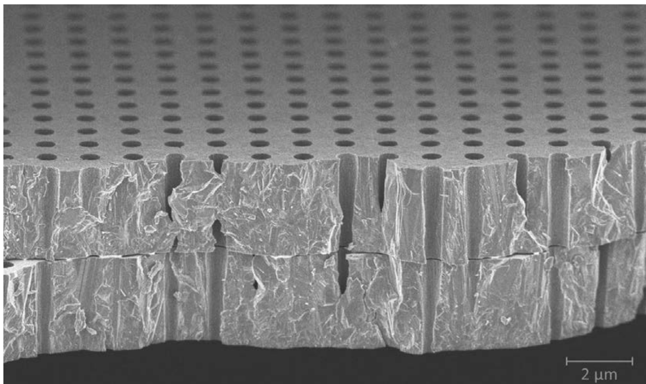
(2) Rasterelektronenmikroskopie-Aufnahme einer mikrostrukturierten Silizium-Membran zur Herstellung von Mikrobrennstoffzellen. Quelle: IMS CHIPS
