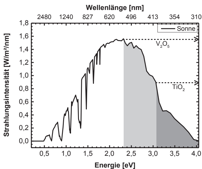
(3) Spektrum des Sonnenlichtes und durch \text{TiO}_2 oder \text{V}_2\text{O}_5 theoretisch nutzbarer Spektralbereich.
