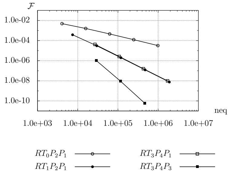
(11) Konvergenz des Funktionalwerts verschiedener Interpolationsordnungen für die regularisierte Nischenströmung für Re = 400 . Hierbei bezeichnet „neq“ die Anzahl der Gleichungen des zu lösenden Systems.
