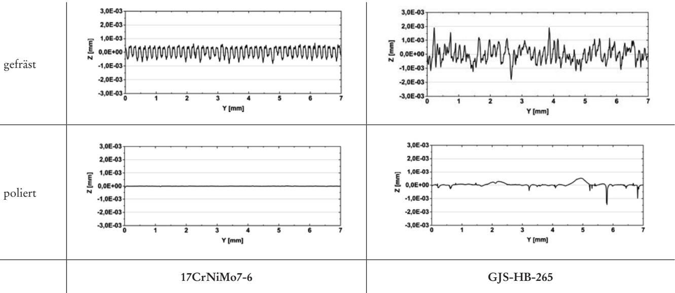
(3) Profilschnitte der gefrästen und polierten Oberflächen. Quelle: D. Stickel, A. Fischer, The influence of topography on the specific dissipated friction power in ultra-mild sliding wear: Experiment and simulation, Tribology International, 91 (2015) 48-59.
