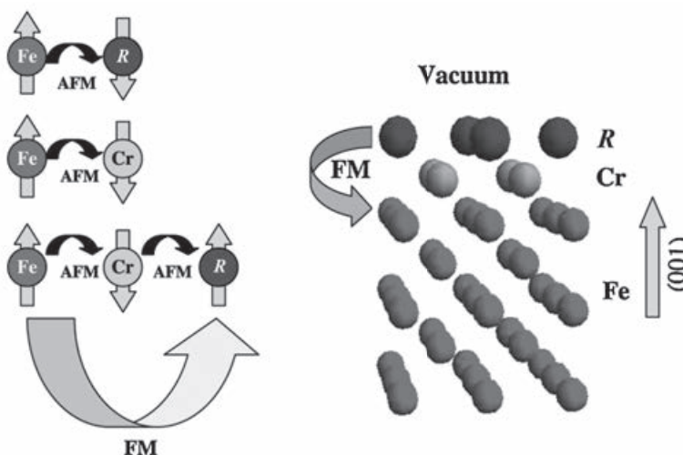
(7) Links: schematische Darstellung der magnetischen Wechselwirkungen zwischen dem Seltenen Erd Metall (R) und den Übergangsmetallen Eisen und Chrom. Rechts: Struktur der entsprechenden Schichtsysteme.
