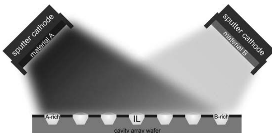
(5) Prinzip des Co-Sputterns in ionischen Flüssigkeiten zur Erzeugung hochreiner Legierungsnanopartikel.
