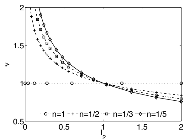
(12) Darstellung der Viskositätsfunktion für verschiedene Fließindizes n . Dilatanz (links) und Strukturviskosität (rechts).
