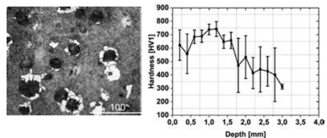
(6) Gefüge und Härteprofil des flammgehärteten GJS-HB-265.
