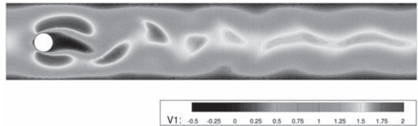
(8) Kármánsche Wirbelstraße.
